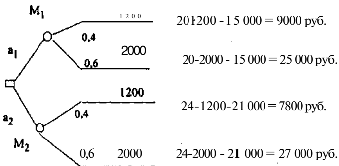
Рис. 2.2. Дерево решений
